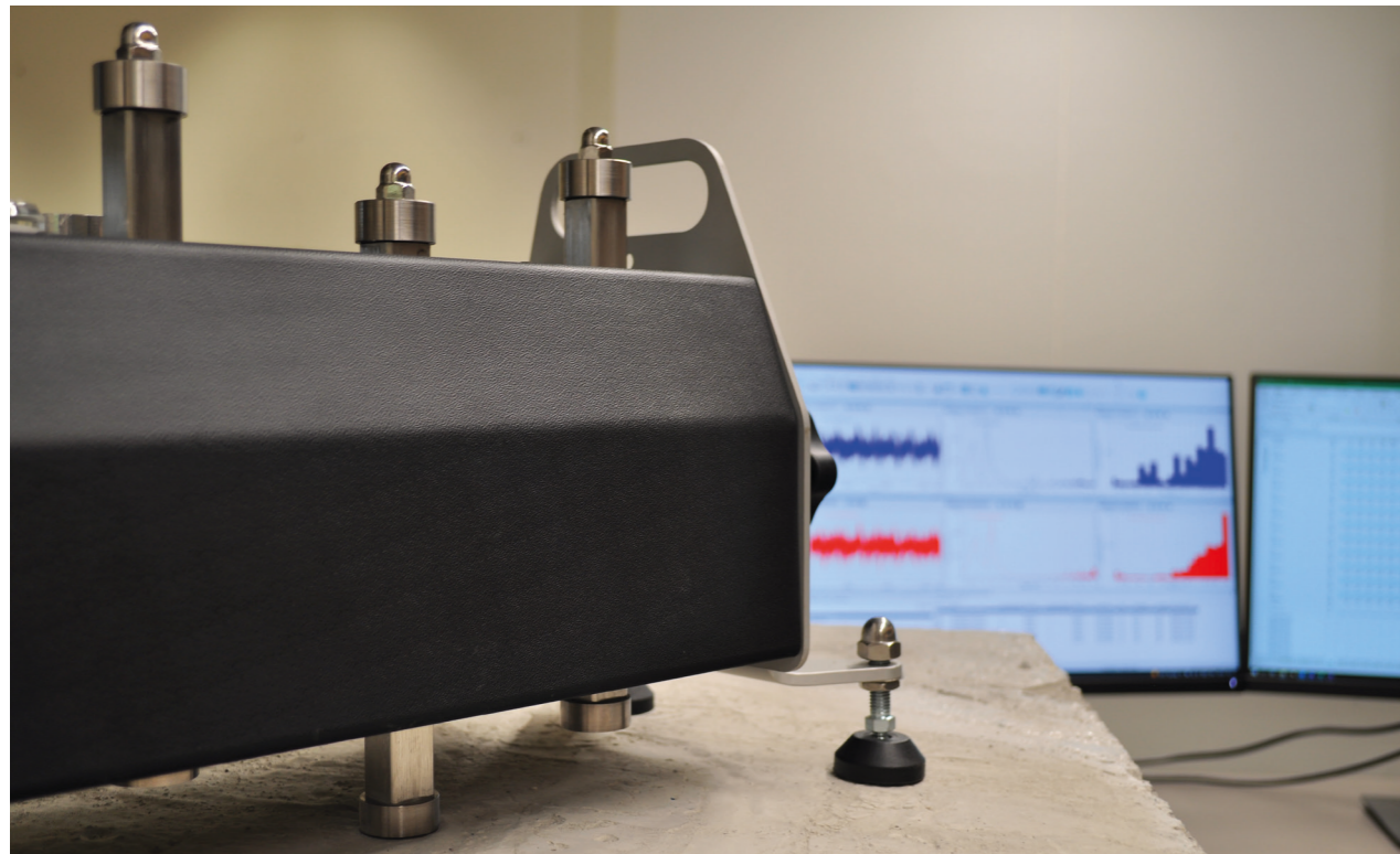
Als Trittschallquelle dient ein Norm-Hammerwerk.
